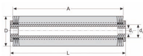
Schemat szczotki składanej
